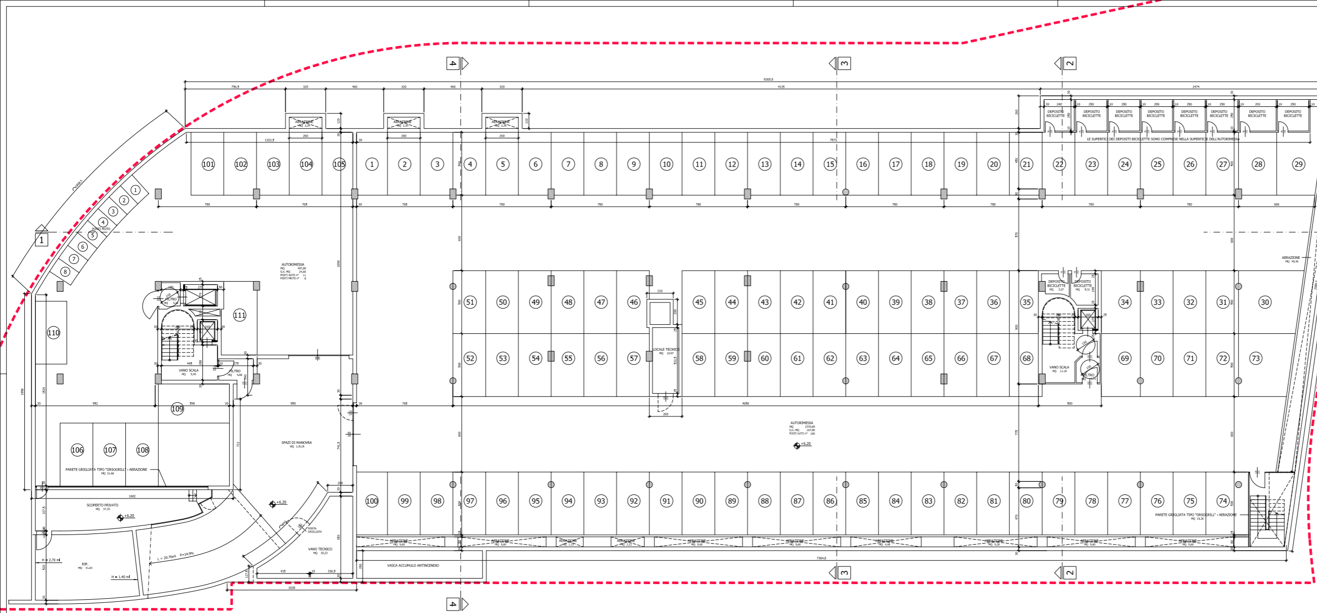
PIANTA PIANO INTERRATO (Q.ta +6.20)
